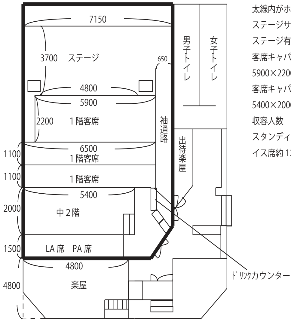
平面図 (単位mm)
