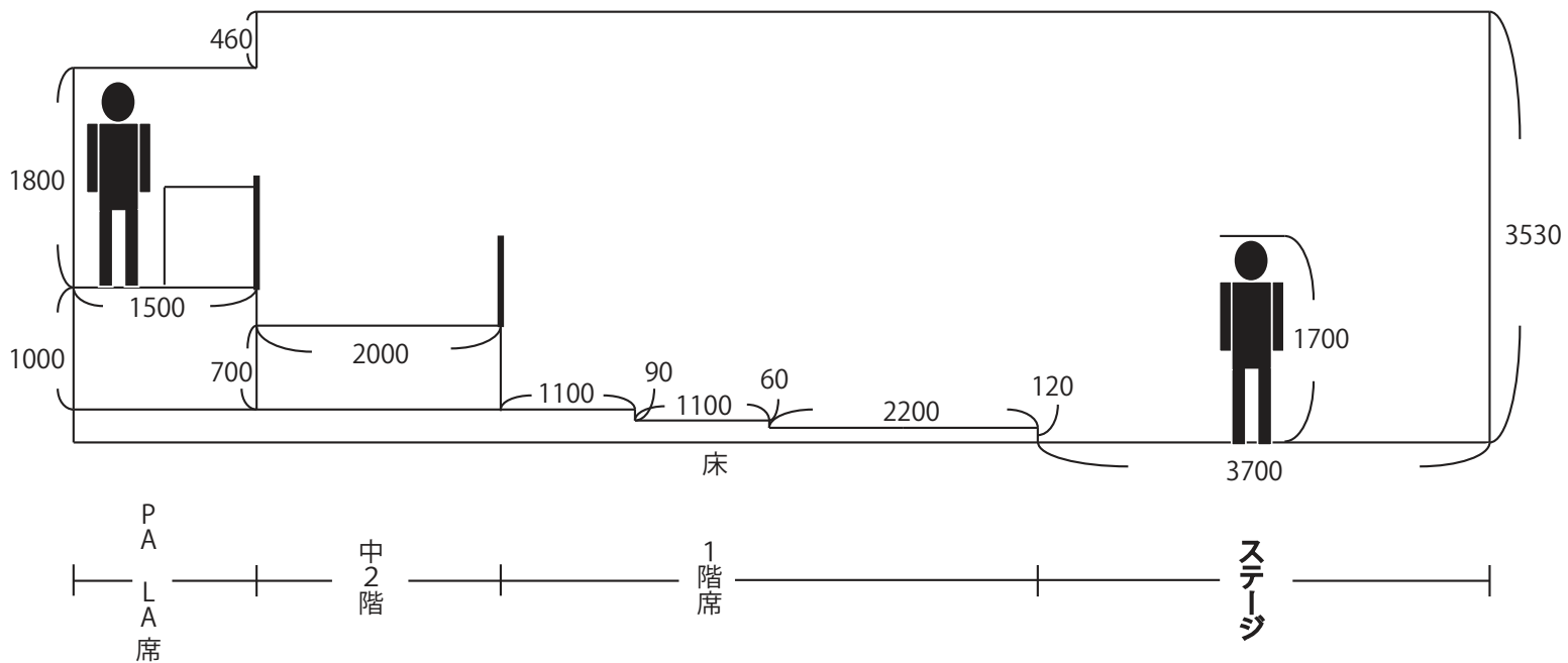
立面図 (単位mm)
